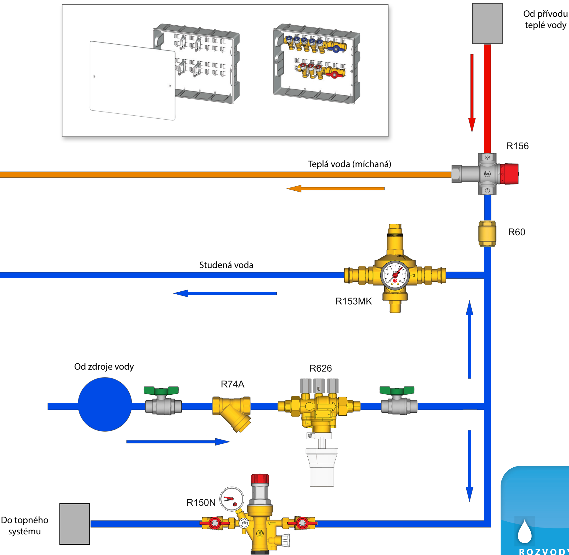
Modulové rozdělovače pro sanitární vodu se skříní
