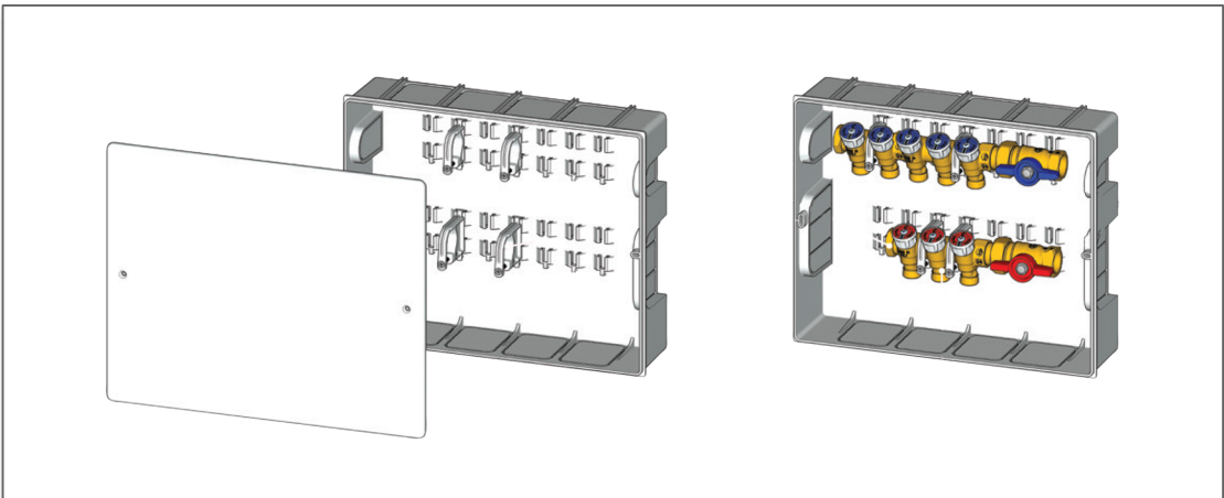
Modulové rozdělovače pro sanitární vodu se skříní
