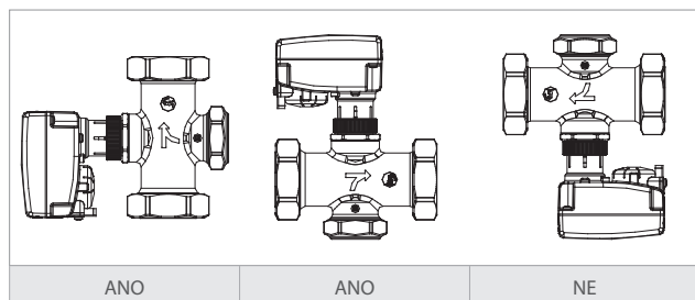
Možné pozice montáže motoru K281
